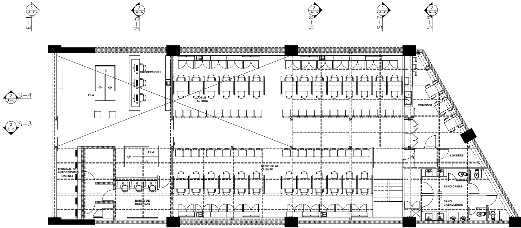
1 PLANTA ARQ. AMUEBLADA PRIMER NIVEL A-3 ESCALA 1:75
