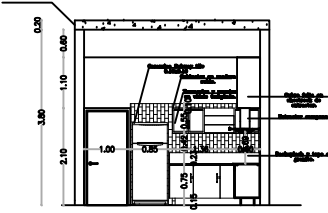
CORTE A-A
