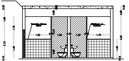
CORTE B-B
