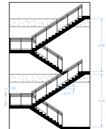
D4 | DETALLE DE ESCALERA PRINCIPAL A-042 | HORMIGON ARMADO, PISO DE ALTO TRAFICO
