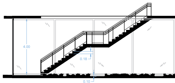
D5 | DETALLE DE ESCALERA AREA SOCIAL A-042 | HORMIGON ARMADO, PISO DE ALTO TRAFICO, JARDINERA SECA AREA CERRADA CON MAMPARA DE CRISTAL
