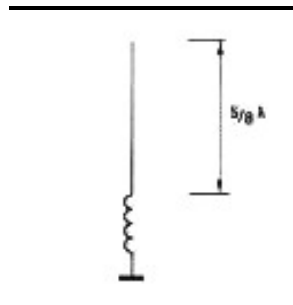
La antena de \frac{5}{8}
