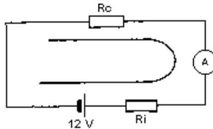
Cálculos con resistencia interna del generador
