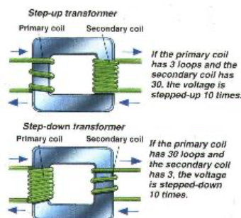
Transformadores y detalles de un transformador
