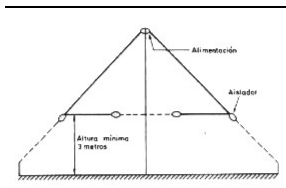
V invertida con las puntas dobladas
