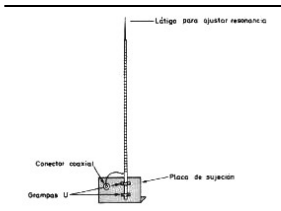
Antena helicoidal
