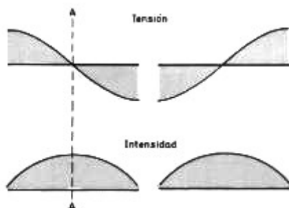
Distribución de corriente y tensión en un dipolo de \lambda
