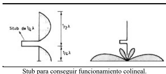
Stub para conseguir funcionamiento colineal.
