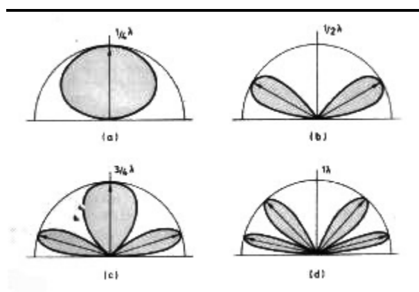
Ángulos verticales de radiación del dipolo para varias alturas.
